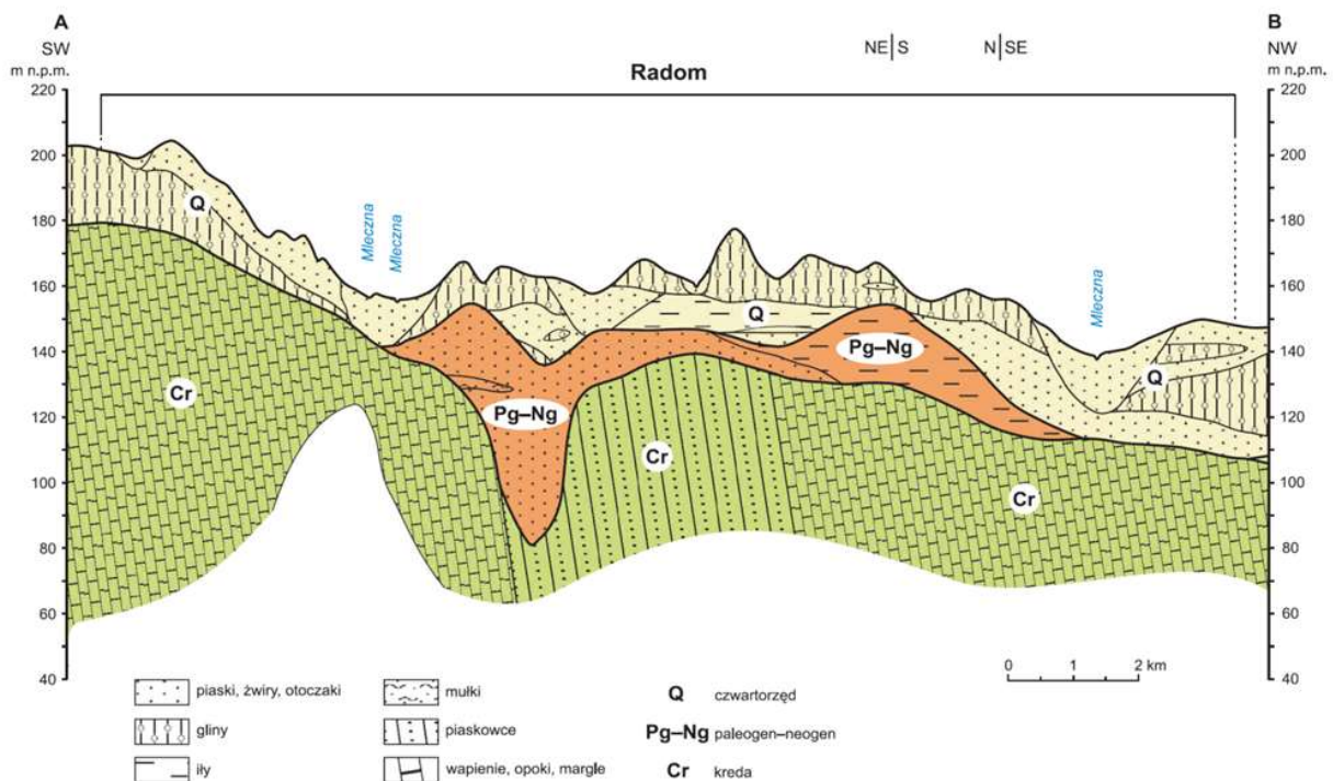
Ryc. 6. Przekrój geologiczny - Radom
