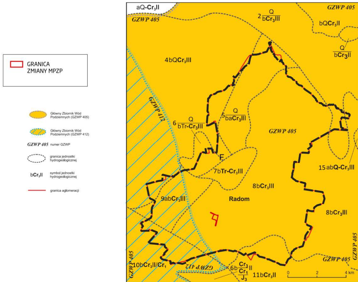
Ryc. 6. Mapa warunków hydrogeologicznych okolic Radomia
