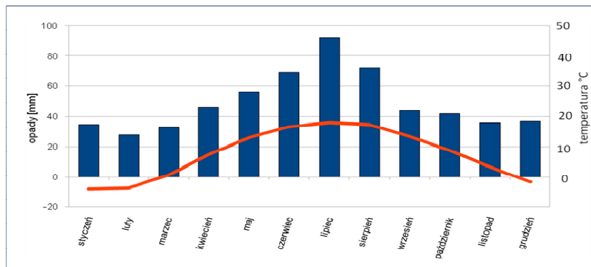
Ryc. 8. Przebieg średnich miesięcznych opadów atmosferycznych i temperatur powietrza na obszarze Radomia w latach 1954-1963.
