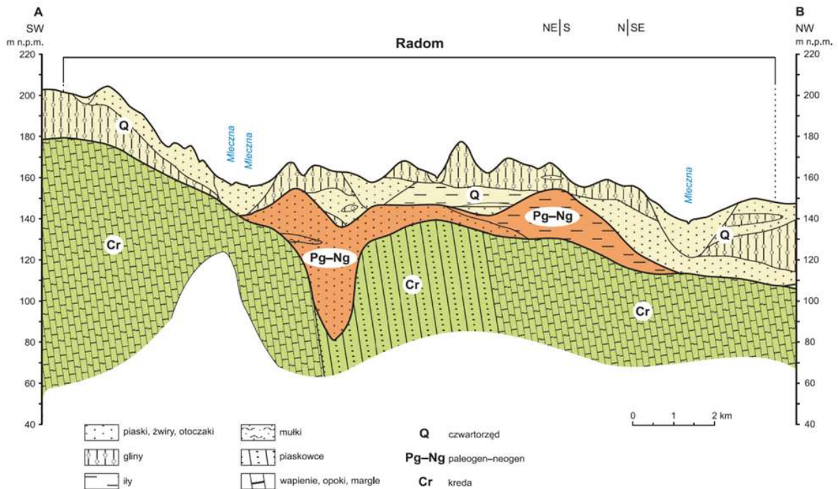
Ryc. 5. Przekrój geologiczny - Radom
