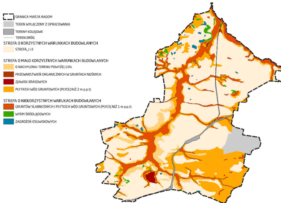
Ryc. 5. Mapa geologiczno-gruntowa
