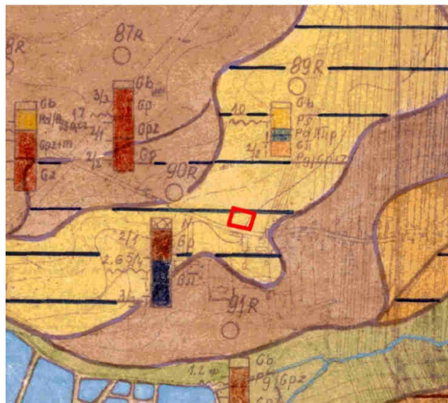
Ryc. 6. Mapa geologiczno-gruntowa
