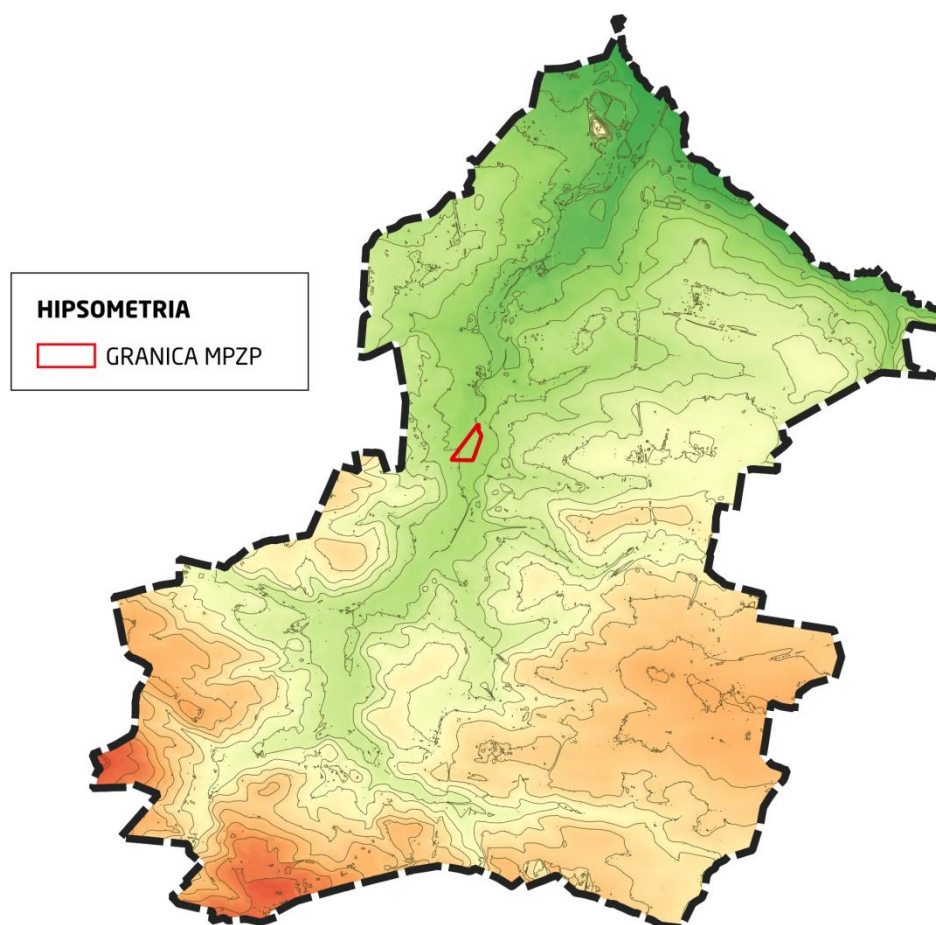
Ryc. 5. Hipsometria (granice zmiany planu oznaczono linią koloru czerwonego)
