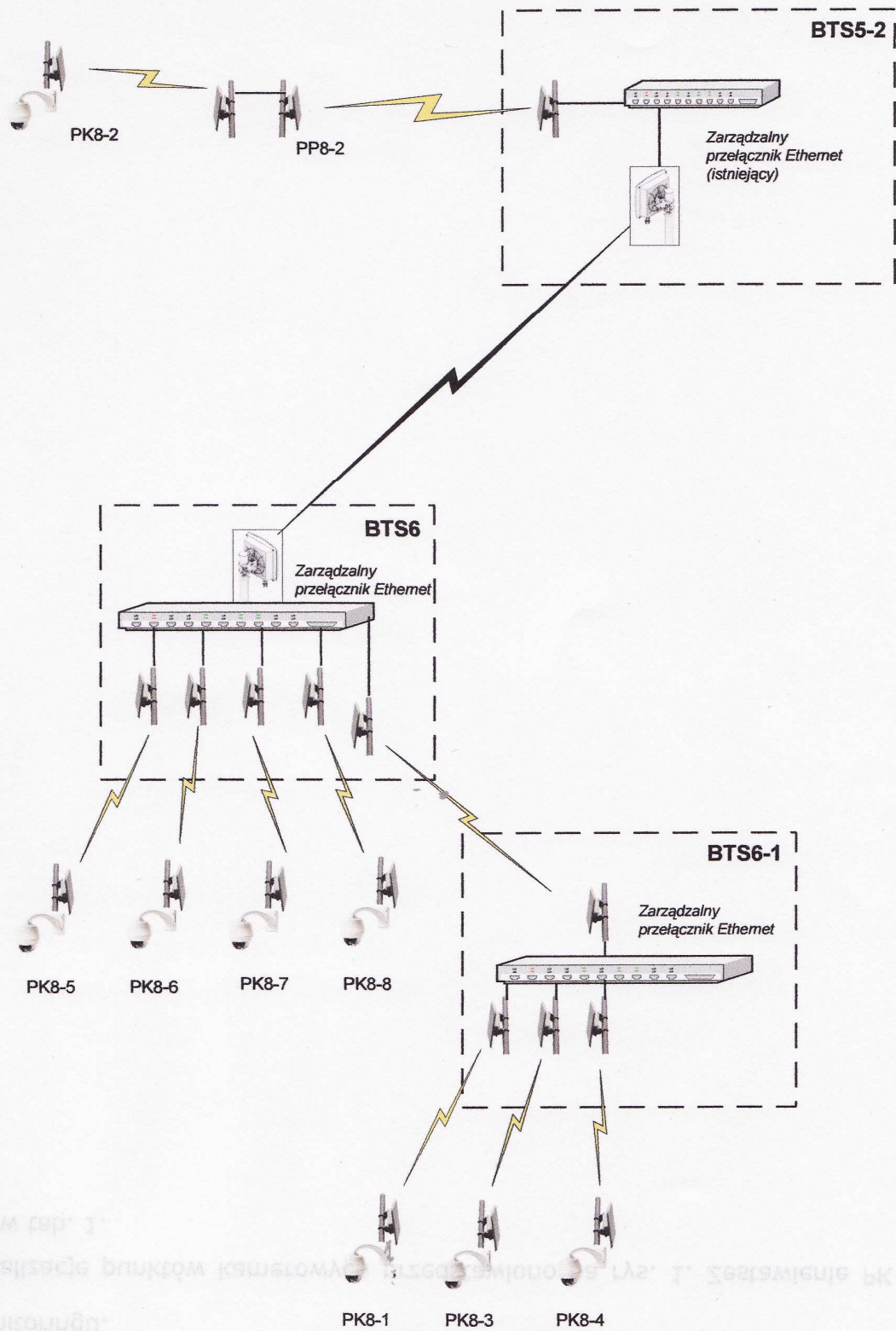
Rys. 2. Schemat logiczny połączeń
